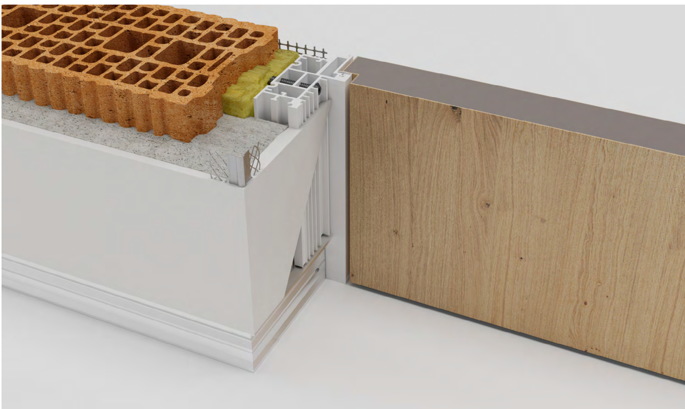
LIBERO 40 - otevírání ven, rubová strana
