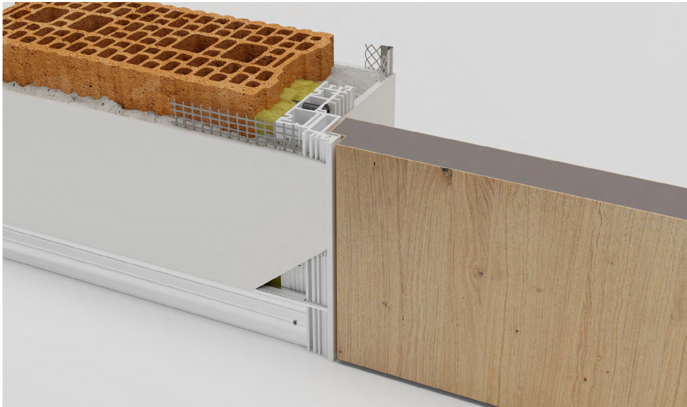
LIBERO 40 - otevírání dovnitř, líčující strana
