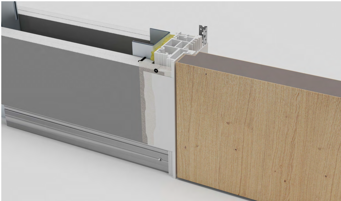
LIBERO 40 - otevírání ven, líčující strana
