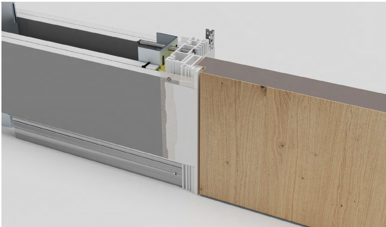
LIBERO 40 - otevírání dovnitř, lícující strana
